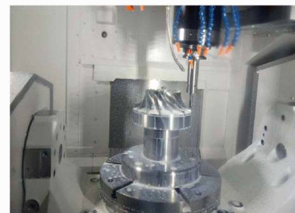
五轴加工机
